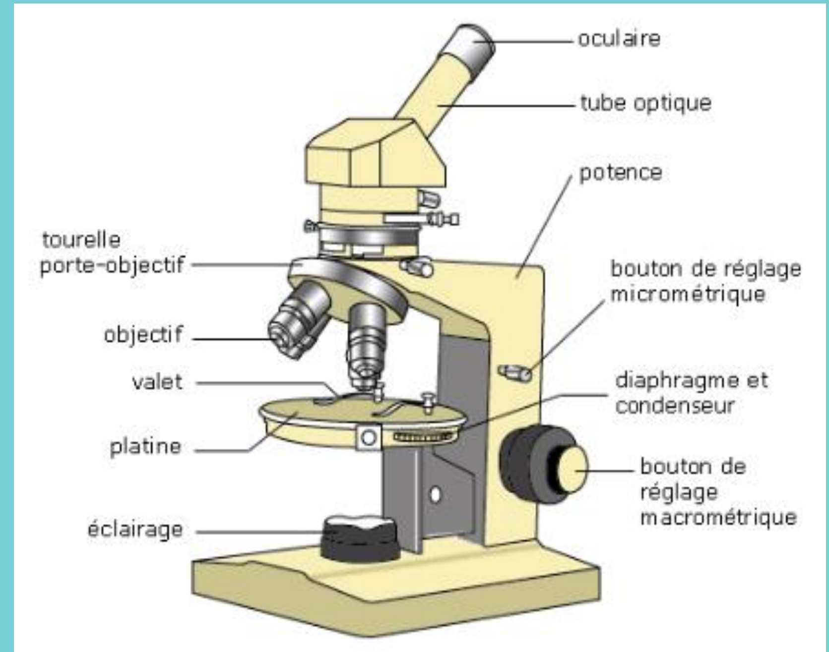
Figure 1 : Description du microscope optique (® Prof Innovant )
